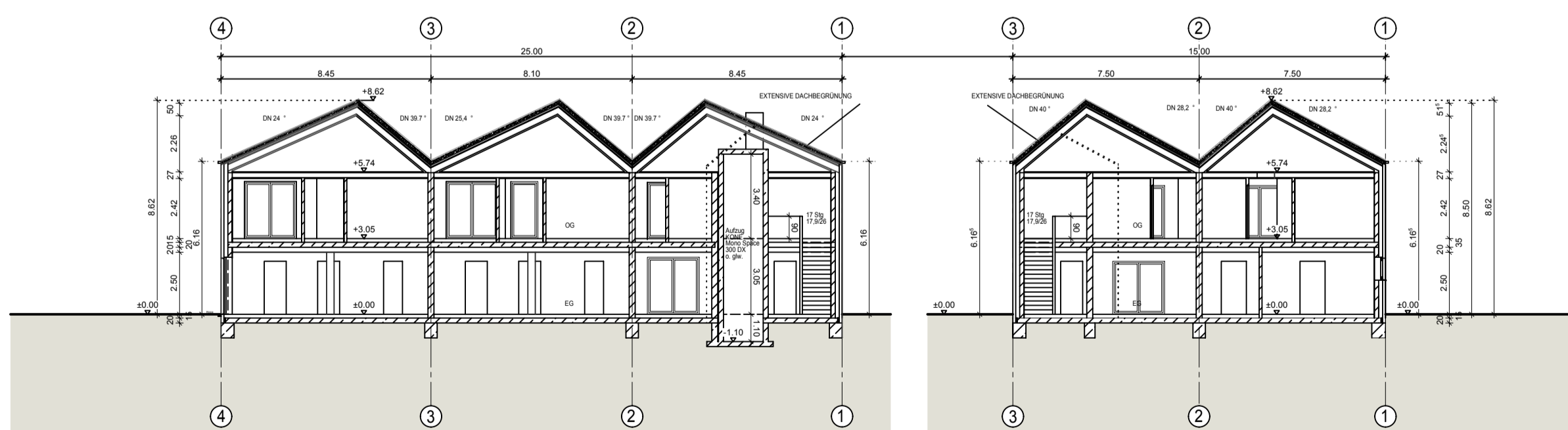
SCHNITTE HAUS 18 + 14
