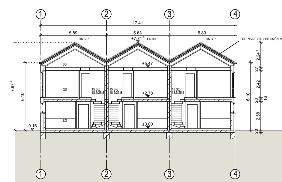
SCHNITT HAUS 16
