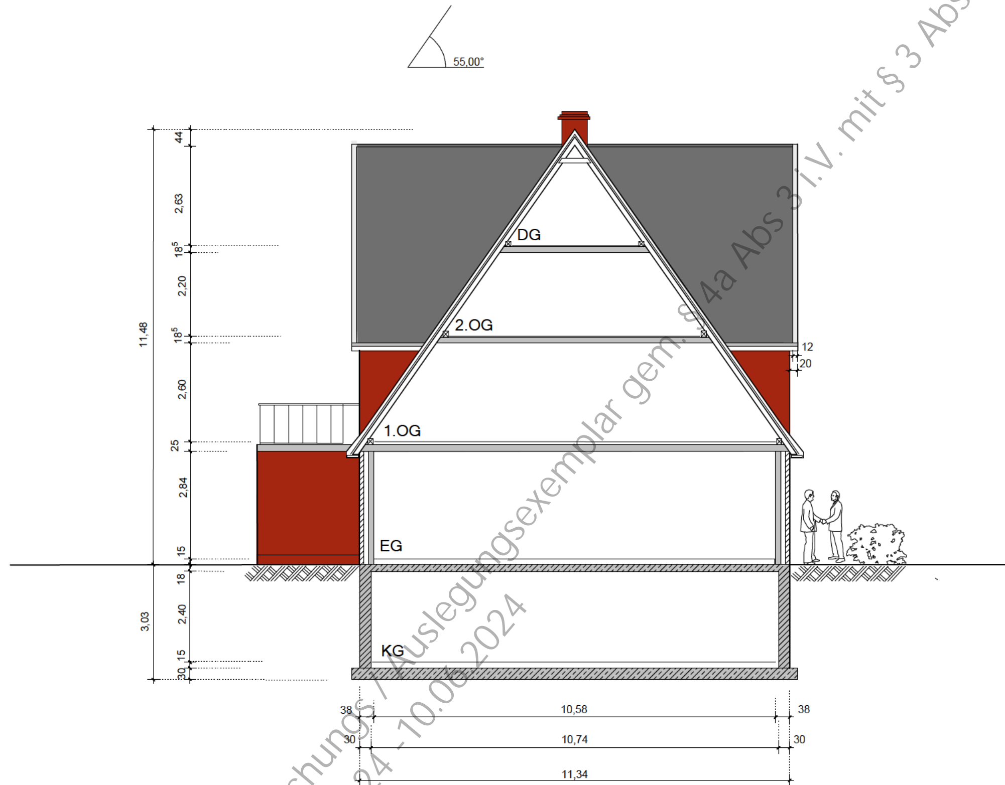
QUERSCHNITT 1-100
