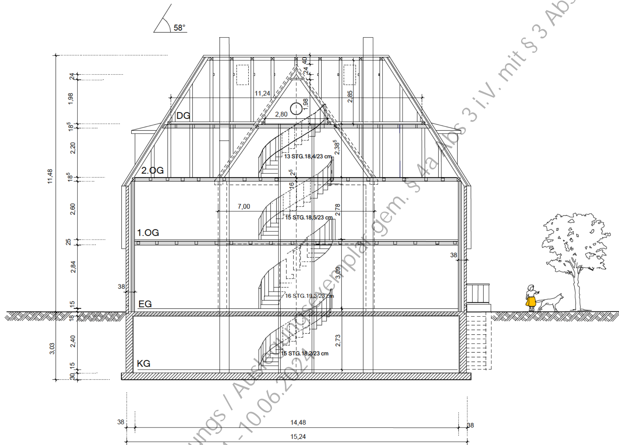
LÄNGSSCHNITT 1-100
