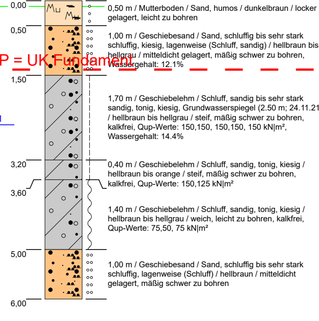
Profil 2 Höhenbezugsniveau (OK SD) = 0,00 m gesetzt
